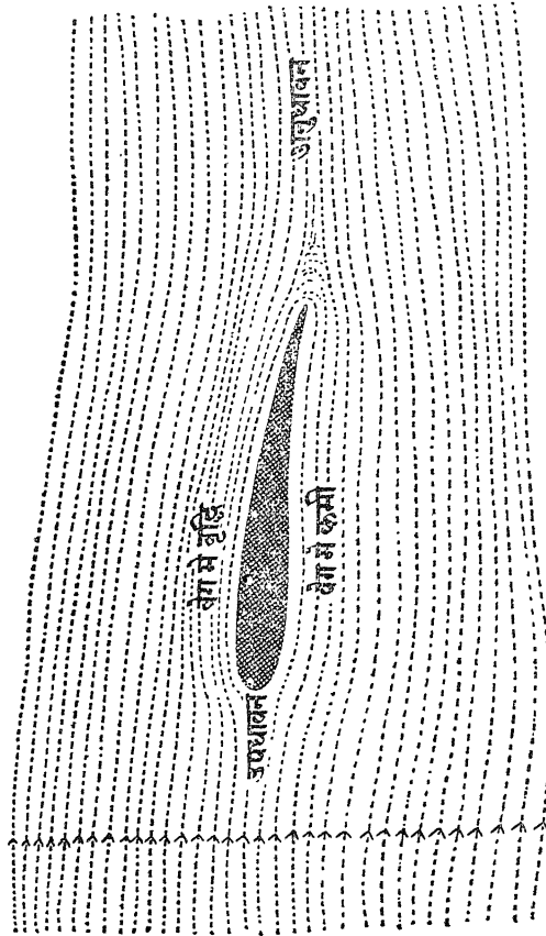
चित्र २५—थोड़े कोण पर झुके पंखकाट पर वायु-प्रवाह।
