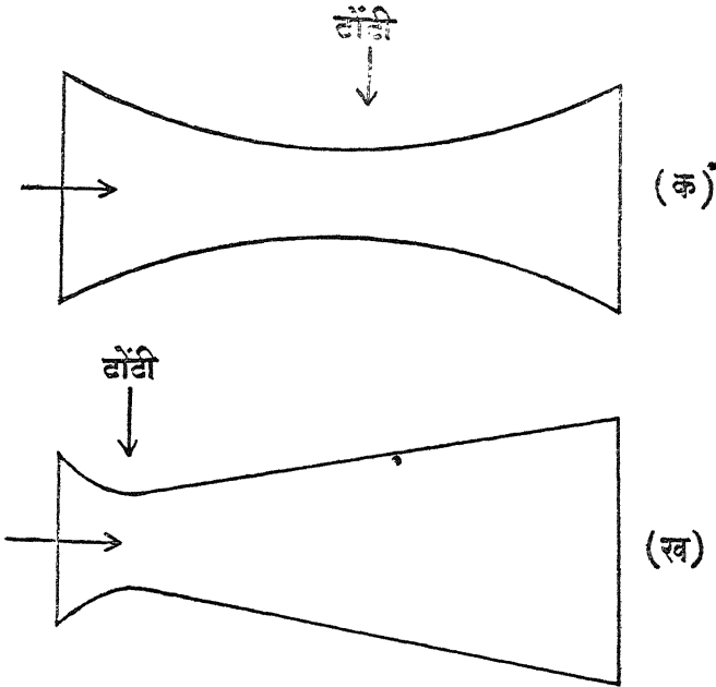
चित्र ६५—अभिबिन्दु-अपबिन्दु दाँटी।
