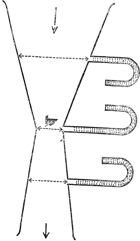
चित्र १७—वेण्ट्री नली ।
