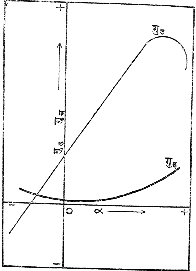
चित्र २९—गुणांक (उद्भार) और गुणांक (वातरोध) के लेखा चित्र।
