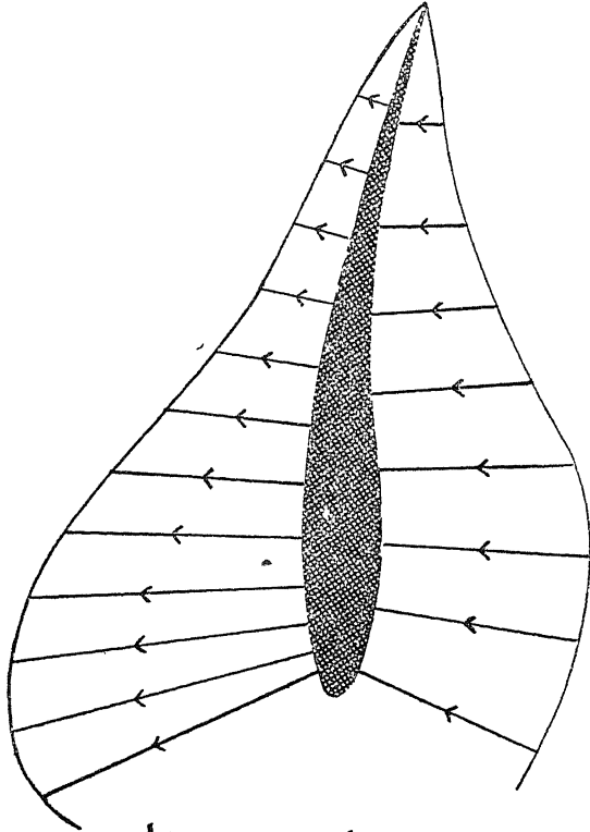
चित्र २२—पंखकाट के चारों ओर दाब वितरण ।
