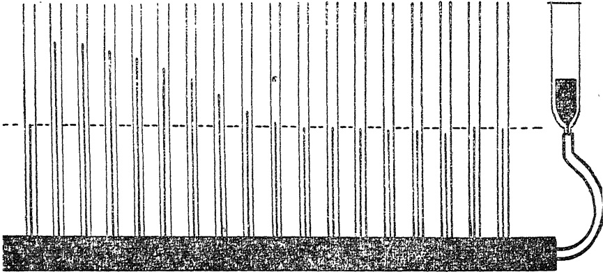
चित्र २७—दाब-मापी।
