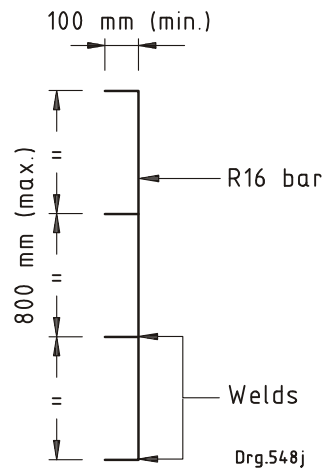
Guide rod detail
